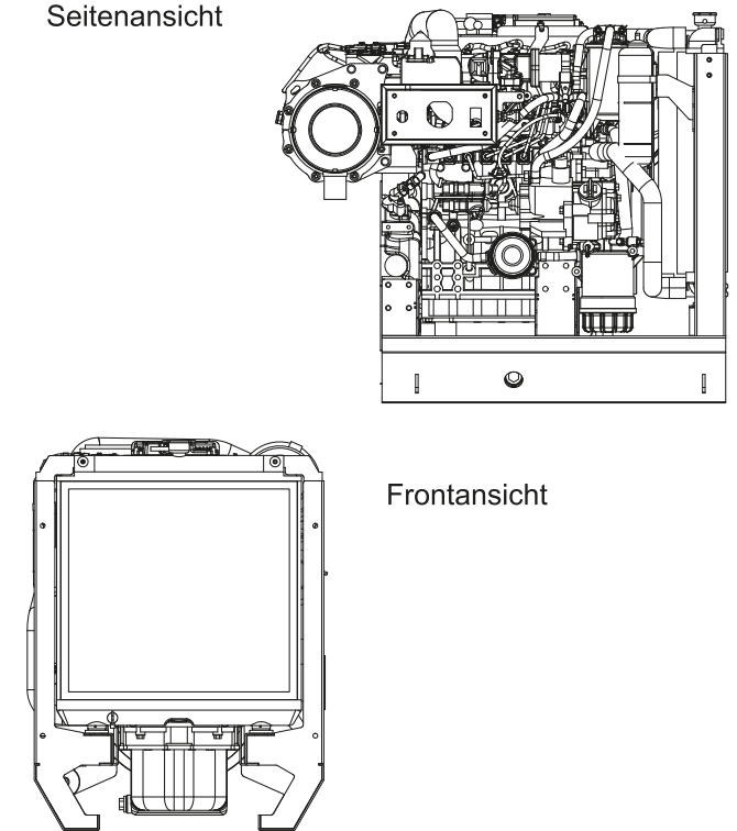
Ansicht ohne Gehäuse Seitenansicht
